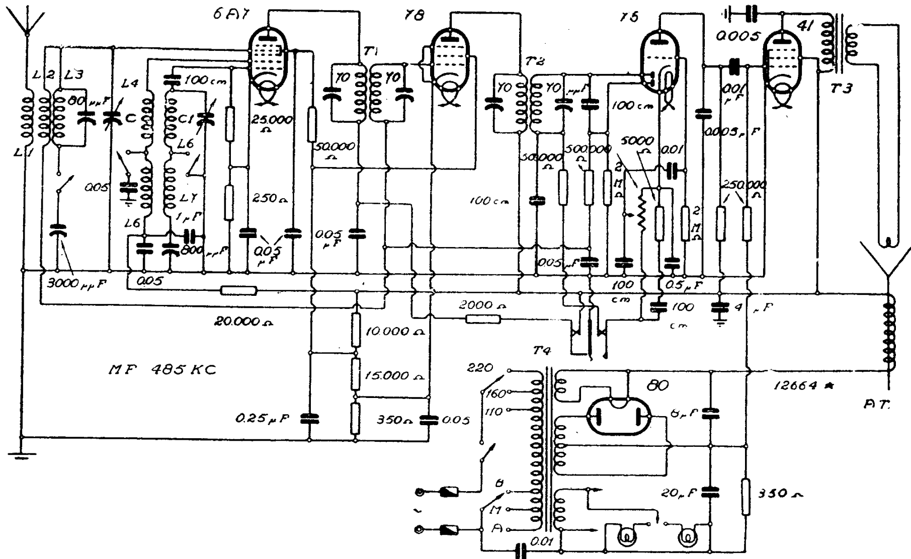
RADIO MARELLI - MOD. «VERTUMNO»
